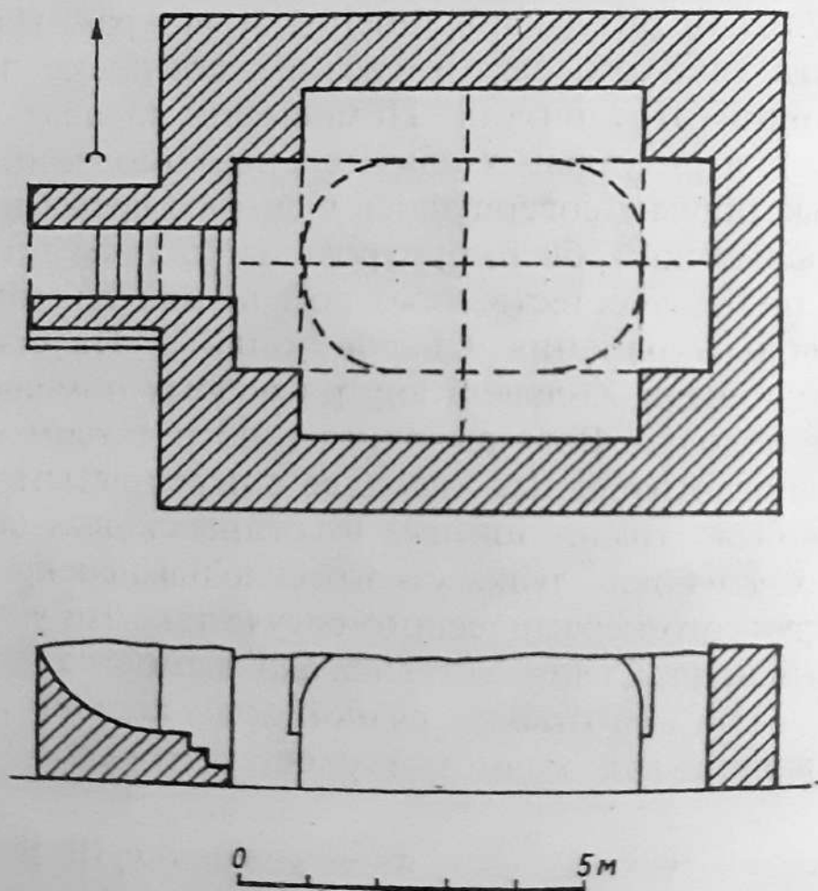
Рис. 28. План Чилля-ханы
