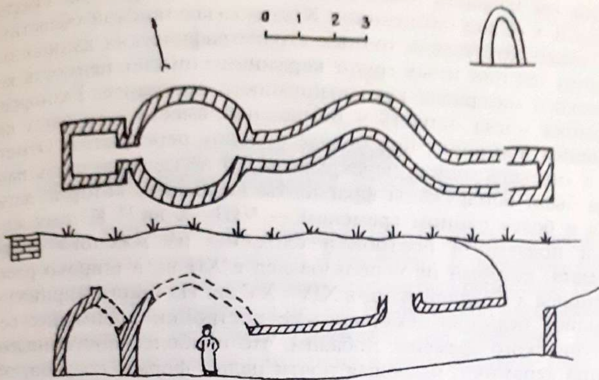
Рис. 29. План Аулие-Кумчик-Ата (по Т. Н. Сениговой)
