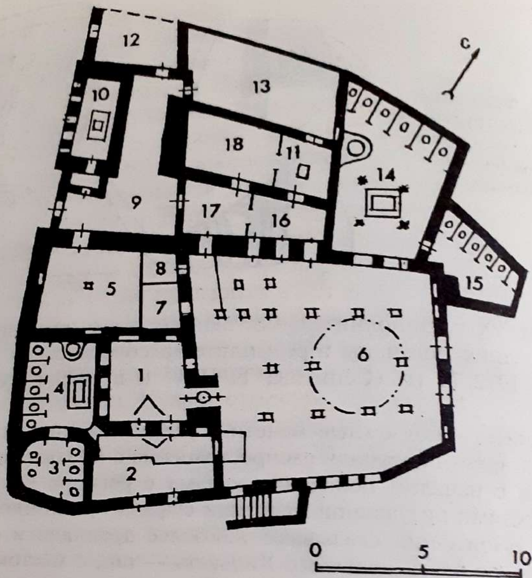
Рис. 27. План макета Большого Хильвета (по Т. Н. Сеиговой)
